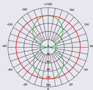
DISTRIBUCIÓN LUMINOSA LIGHT INTENSITY DISTRIBUTION
